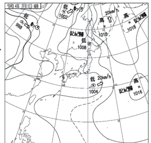
7 月 11 日の天気図 梅雨が明けオホーツク海高気圧は北上、今週は太平洋高気圧が東にそれ、暑さもひと段落。
